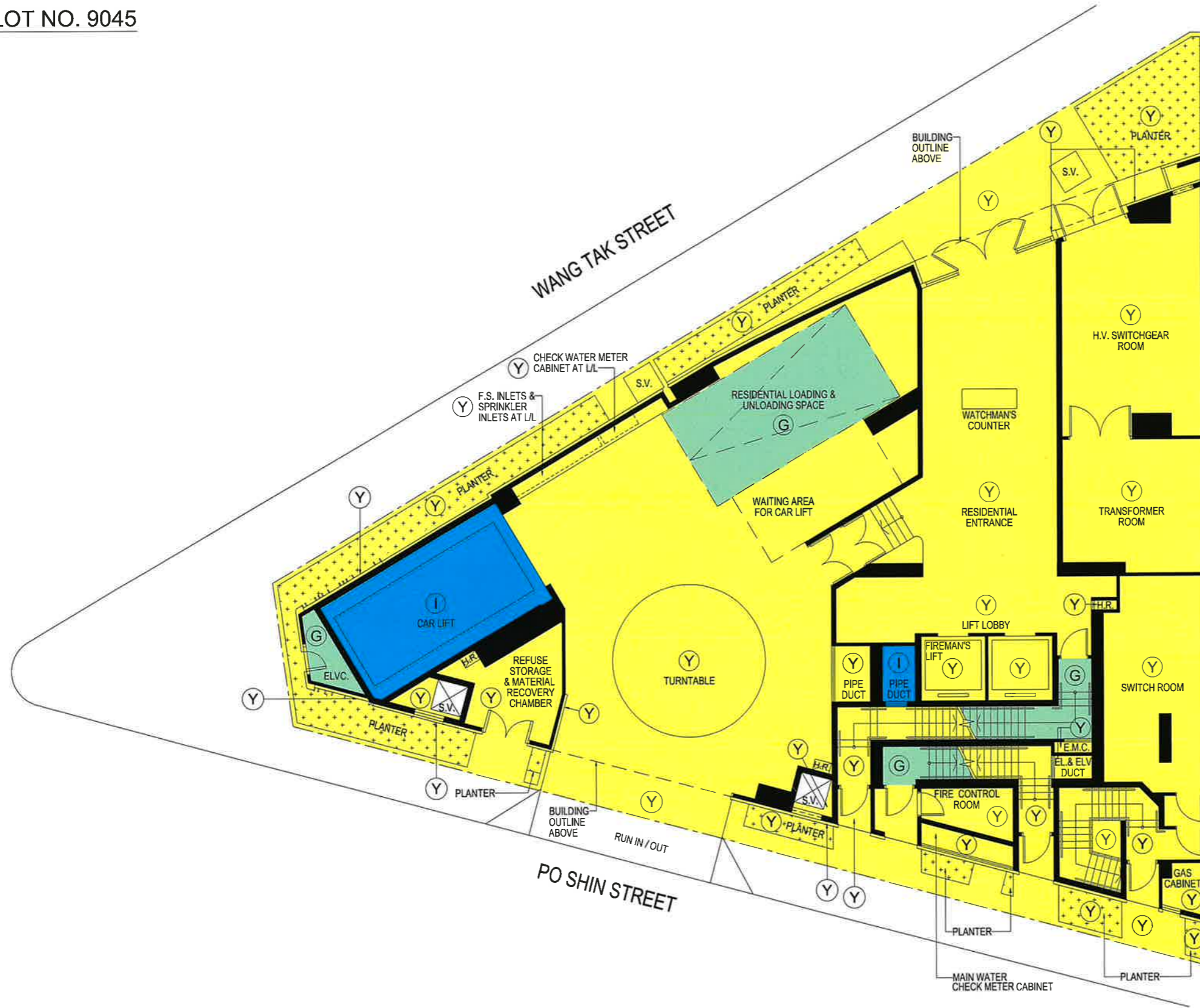
G/F PLAN SCALE : N.T.S.
