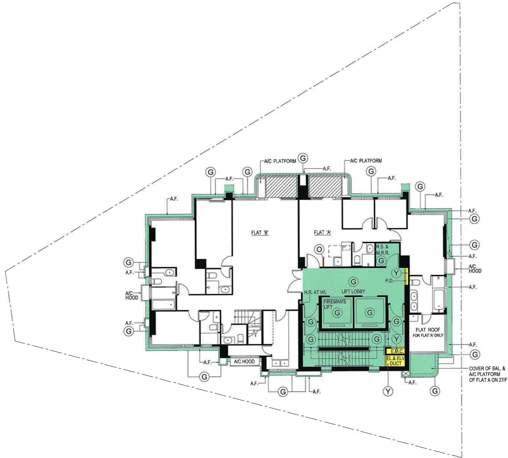
28/F PLAN SCALE : N.T.S.
