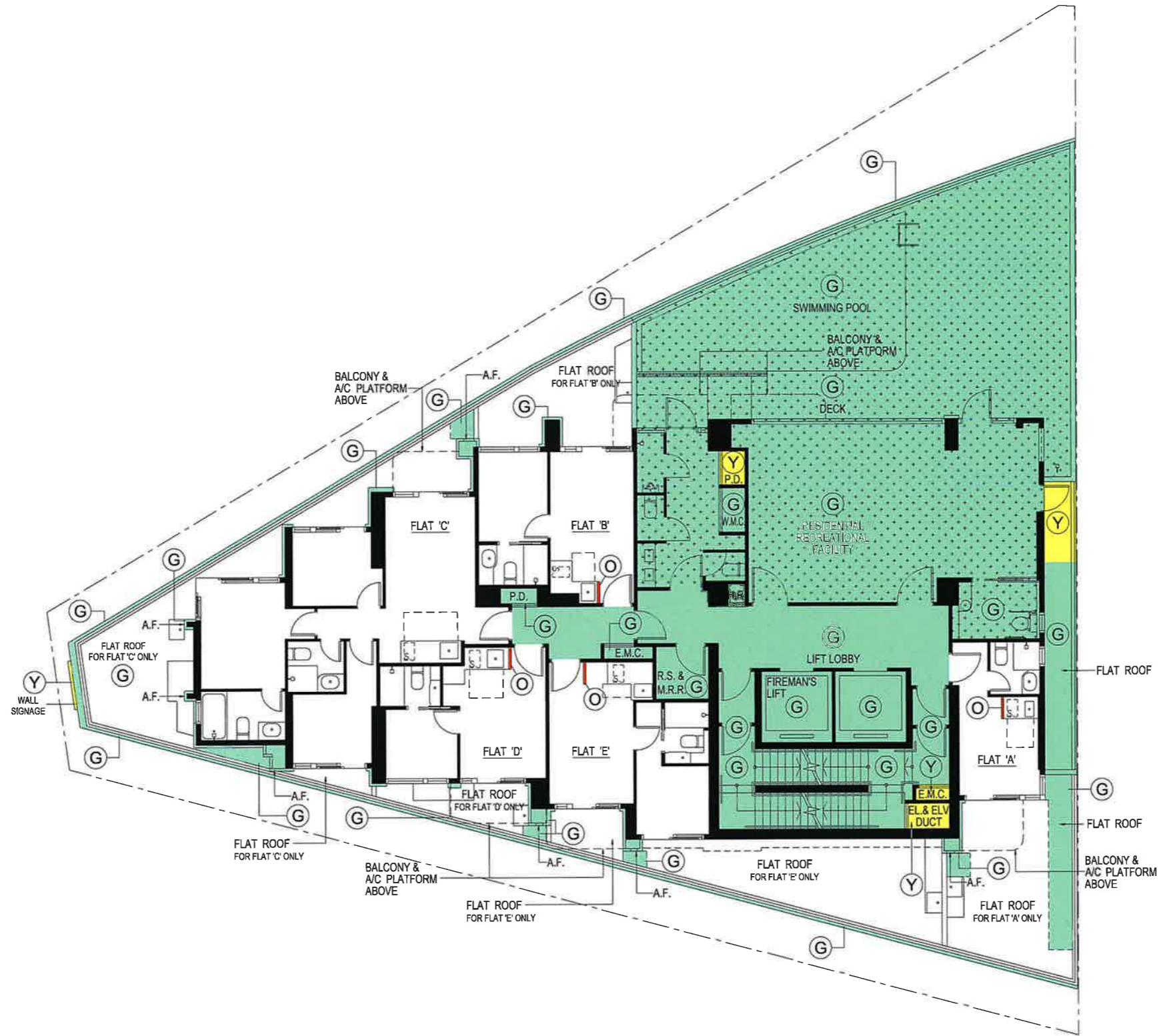
1/F PLAN SCALE : N.T.S.
