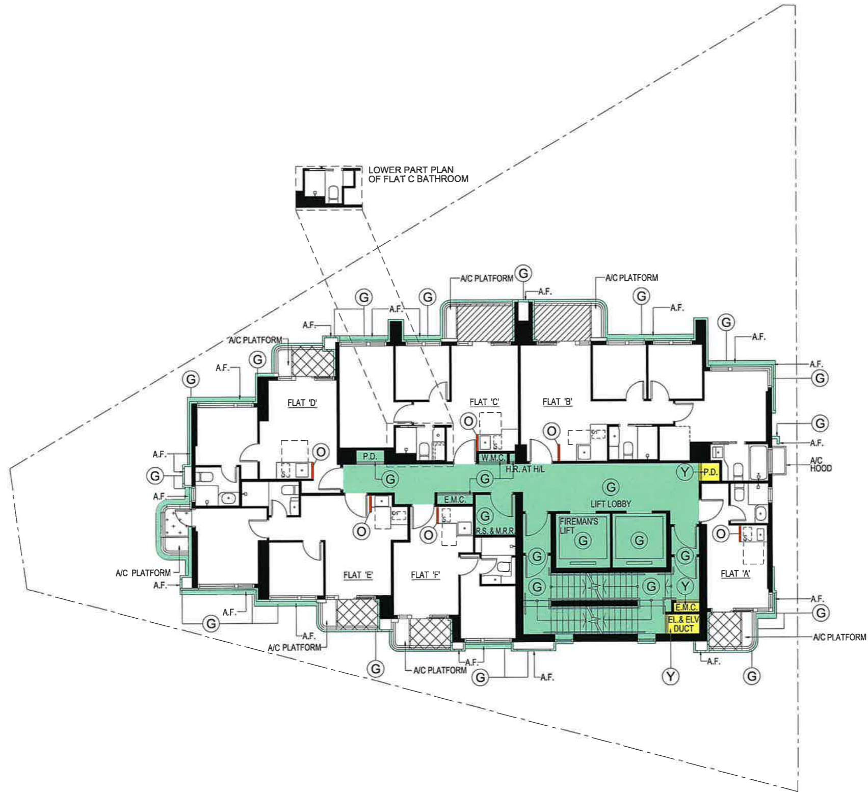
16/F PLAN SCALE : N.T.S.
