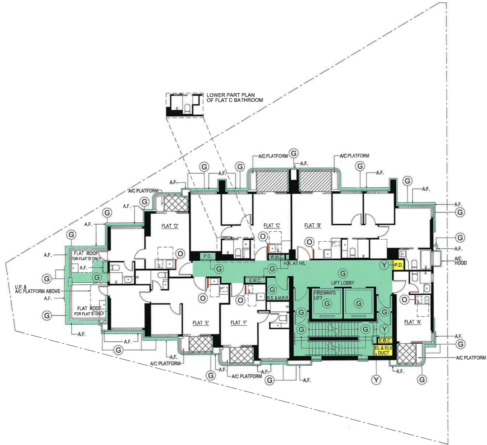
15/F PLAN SCALE : N.T.S.
