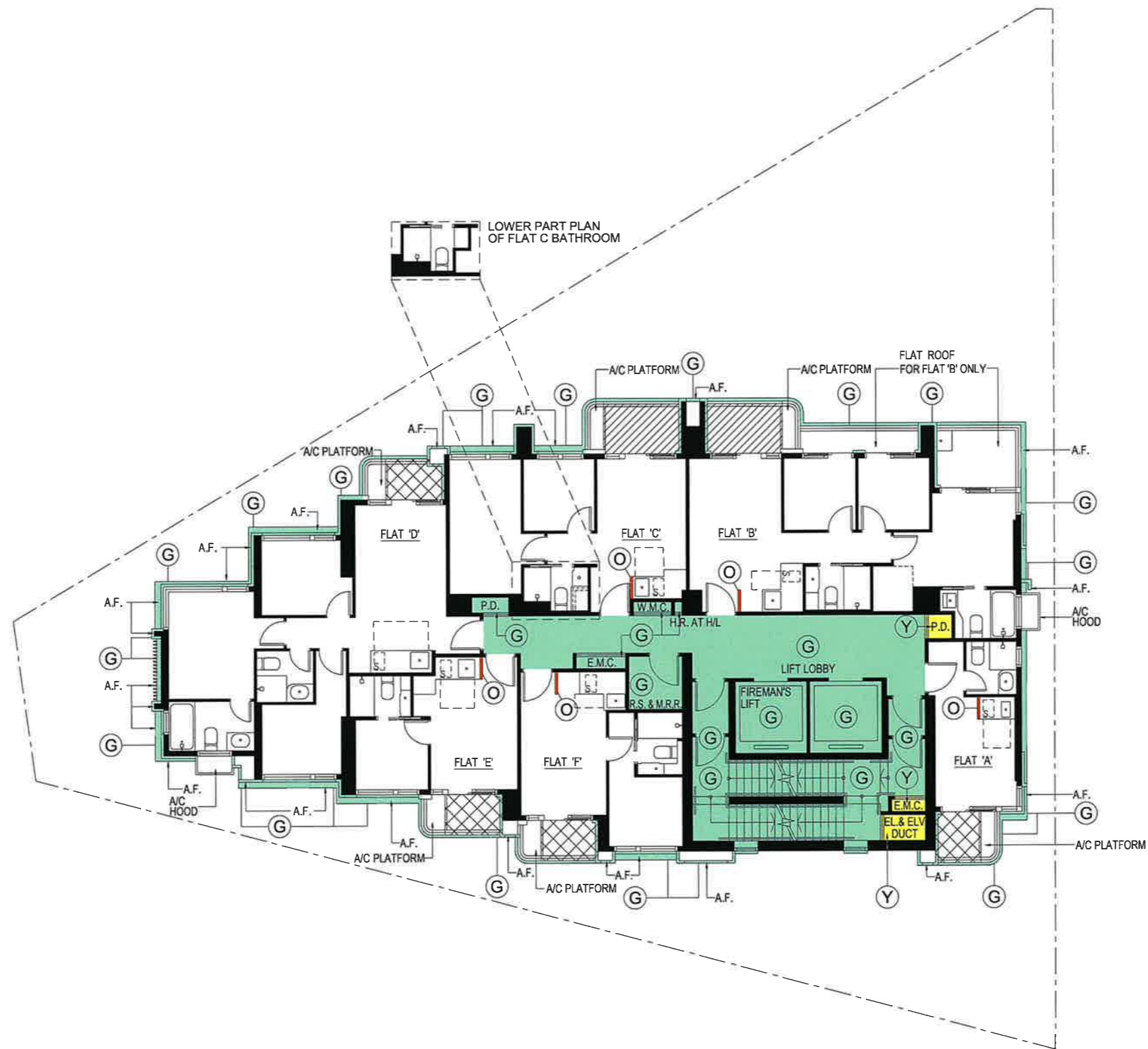
2/F PLAN SCALE : N.T.S.
