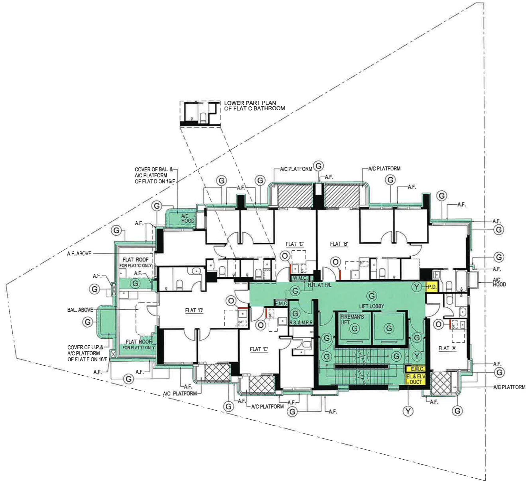
17/F PLAN SCALE : N.T.S.
