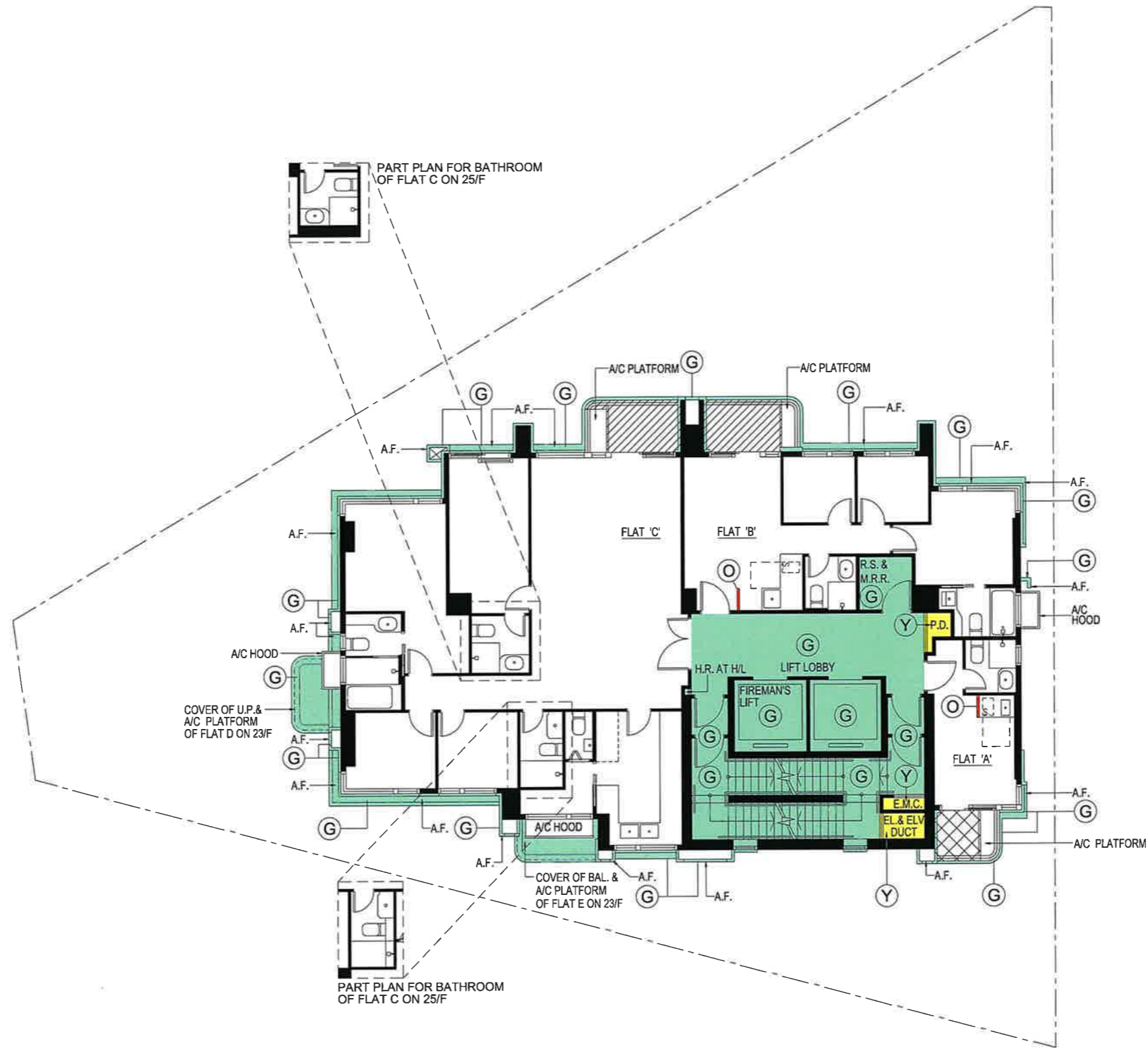
25/F - 27/F PLAN SCALE : N.T.S.
