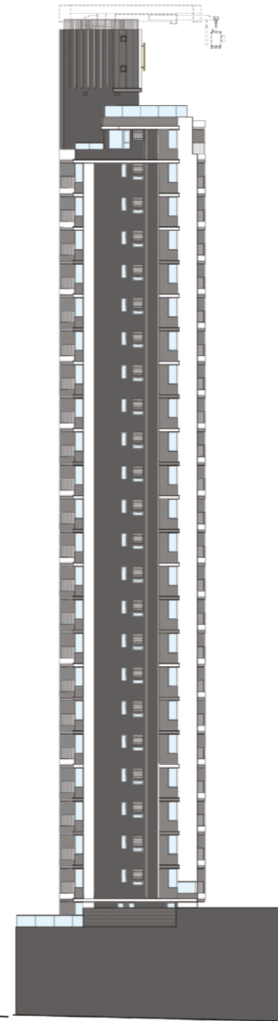
北立面圖 North Elevation
